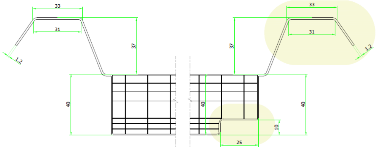
DETALLE LADO A ESCALA 1:1
