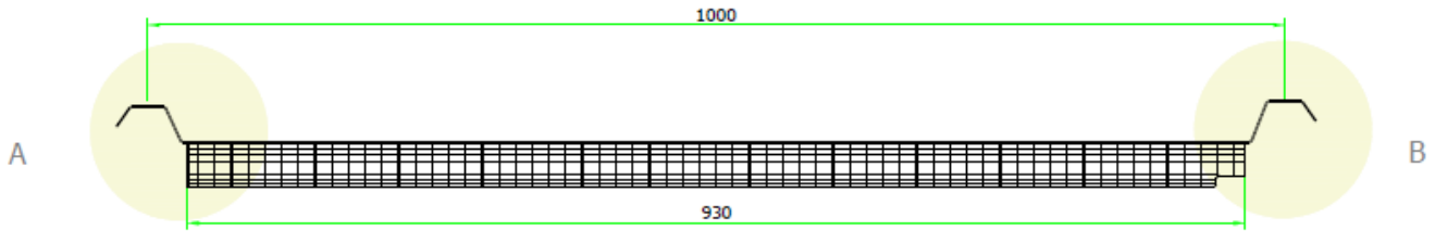
DETALLE GEOMETRÍA COMPLETA ESCALA 1:5
