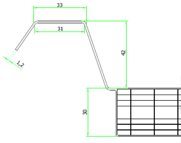
DETALLE LADO A ESCALA 1:1
