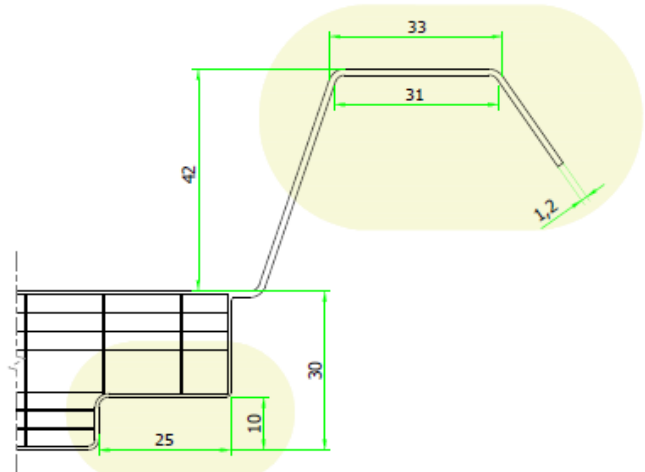
DETALLE LADO B ESCALA 1:1
