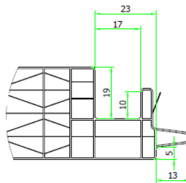
DETALLE GEOMETRÍA COMPLETA ESCALA 1:5
