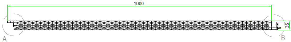
DETALLE GEOMETRÍA COMPLETA ESCALA 1:5
