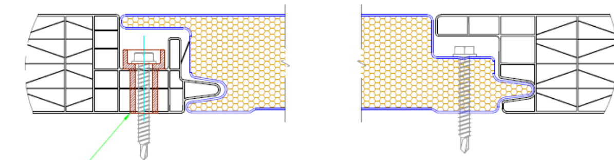
DETALLE ENCUENTRO CON HUURRE FACHADA ESCALA 1:1
