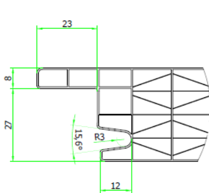
DETALLE LADO A ESCALA 1:1
