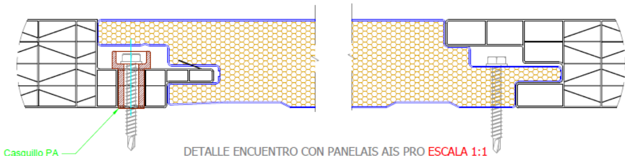
DETALLE ENCUENTRO CON PANELAIS AIS PRO ESCALA 1:1
