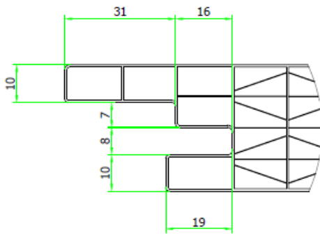
DETALLE LADO A ESCALA 1:1
