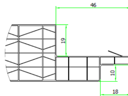
DETALLE LADO B ESCALA 1:1
