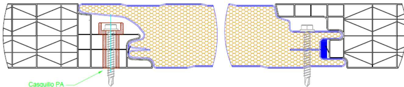
DETALLE ENCUENTRO CON METECNO Superwall 40 ESCALA 1:1
