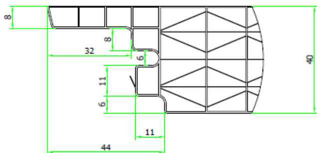
DETALLE LADO A ESCALA 1:1
