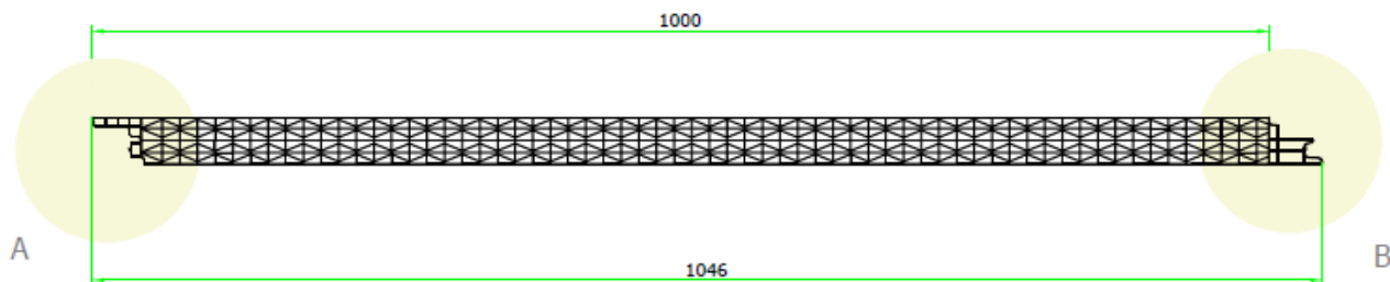
DETALLE GEOMETRÍA COMPLETA ESCALA 1:5
