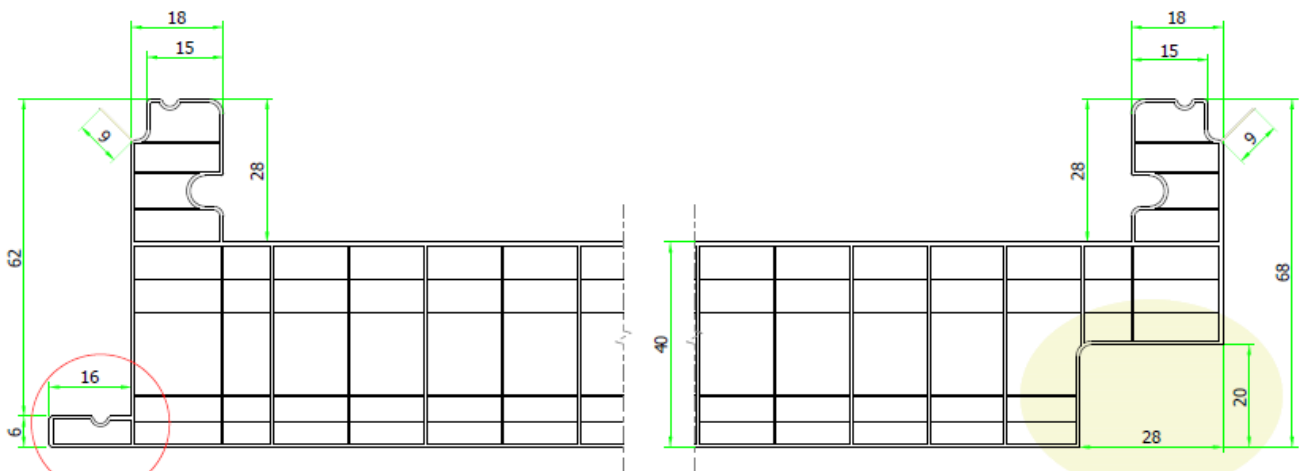
DETALLE LADO A ESCALA 1:1
