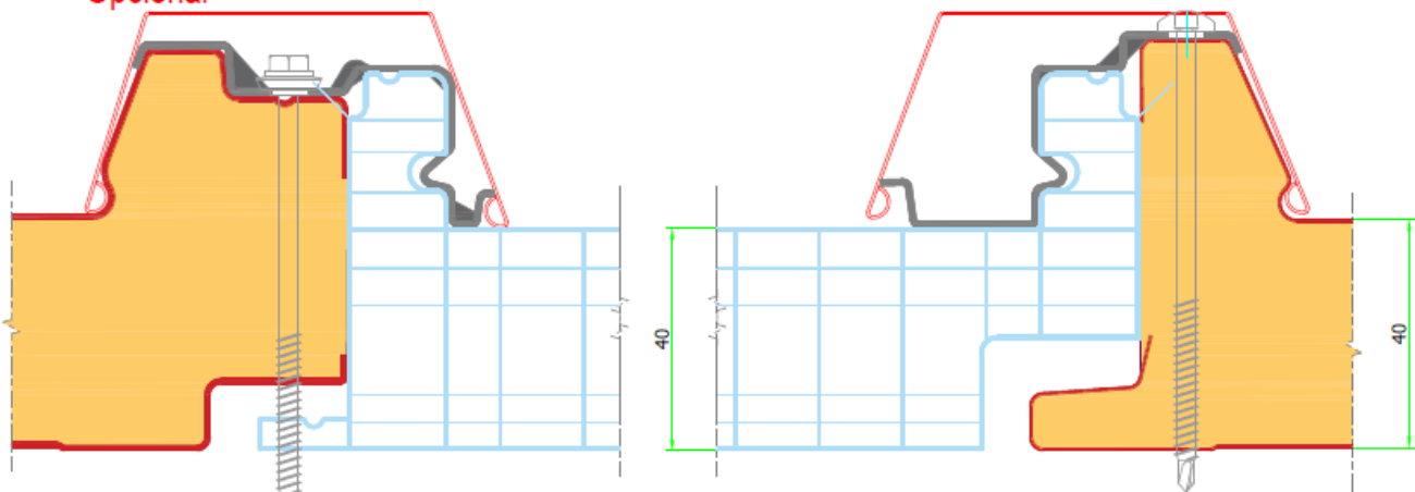
DETALLE DE ENCAJE CON PANEL DE POLIURETANO DE 40mm ESCALA 1:1
