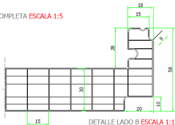
DETALLE LADO B ESCALA 1:1
